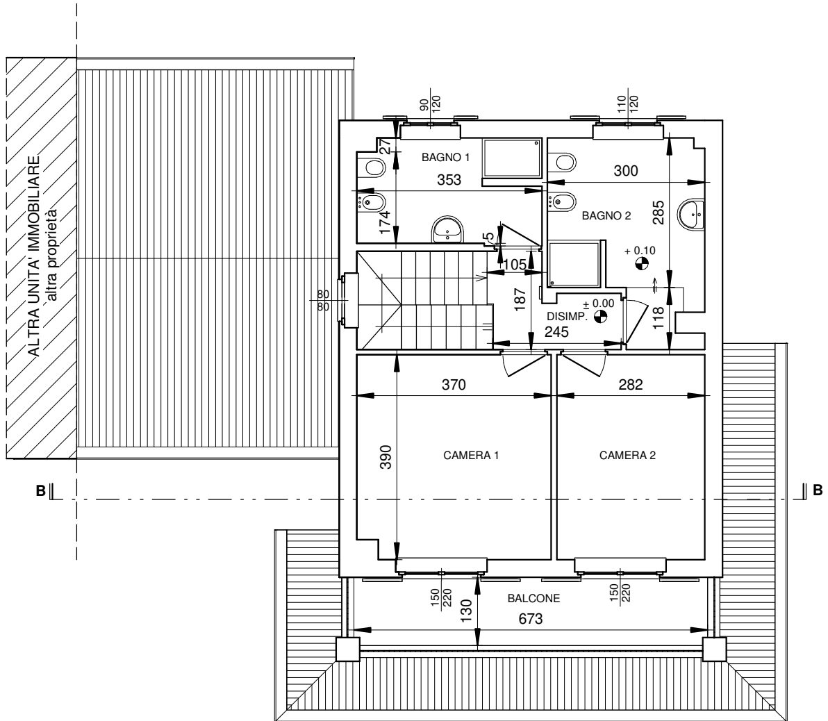
PIANTA PIANO PRIMO - esistente - sc. 1 : 100
